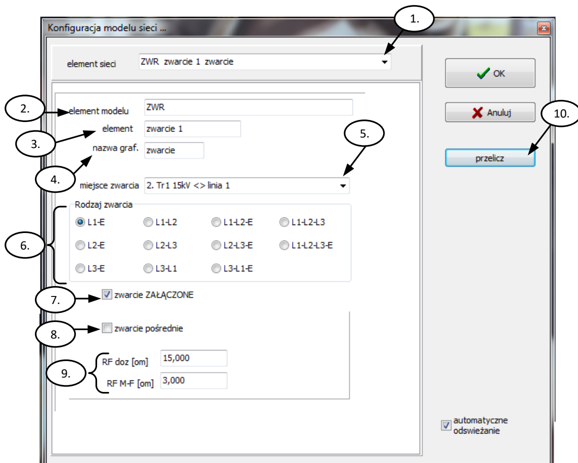
Rys.8.9. Okno edycji parametrów zwarcia
