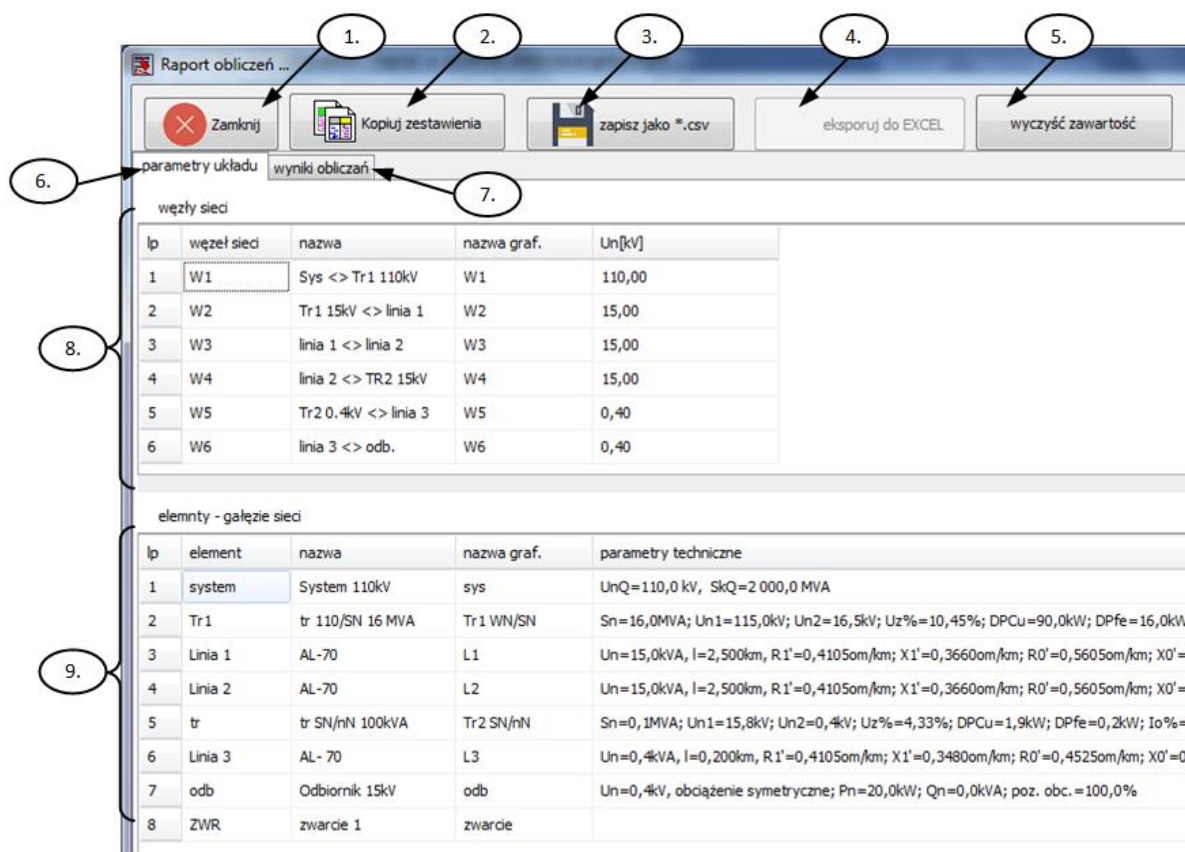
Rys.9.3. Okno raportu obliczeń
