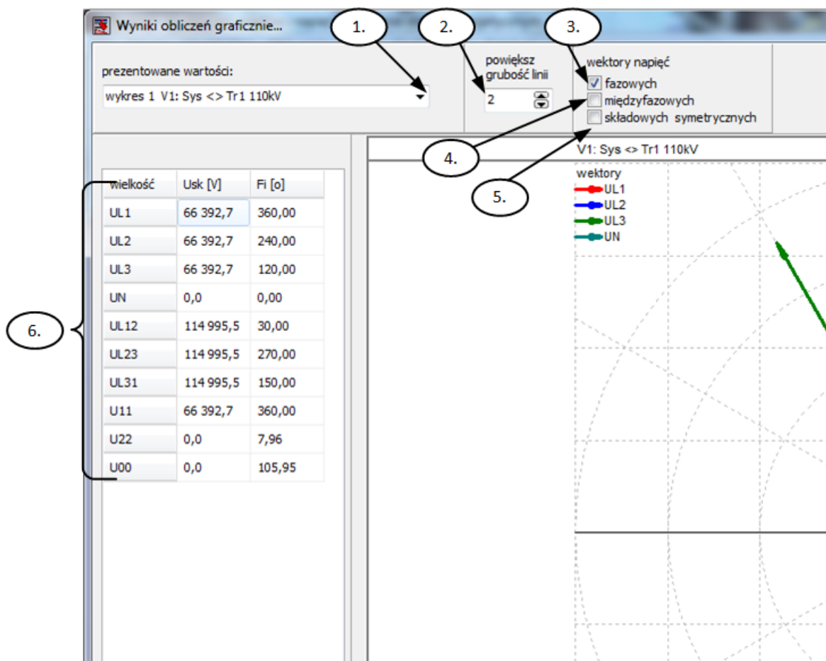
Rys.9.5. Wyniki obliczeń graficznych napięciowych
