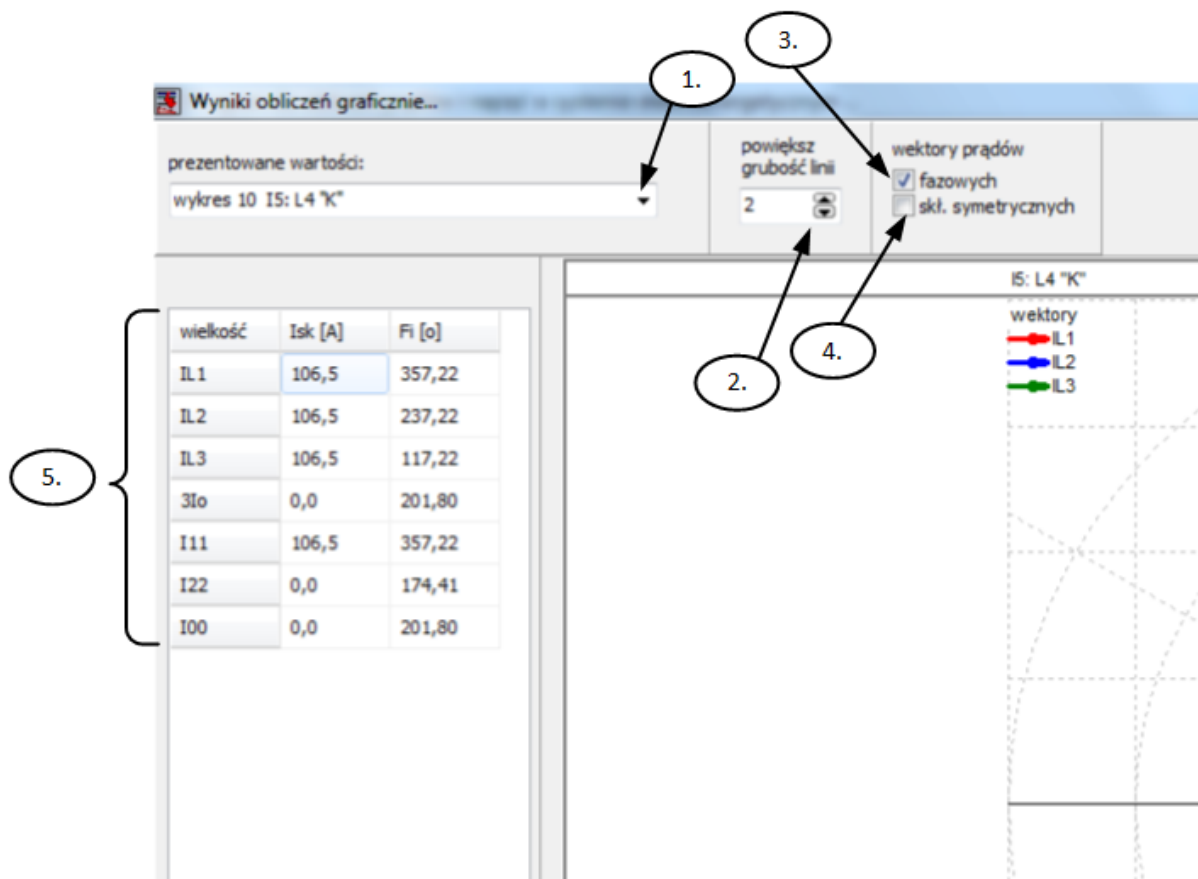
Rys.9.6. Wyniki obliczeń graficznych prądowych
