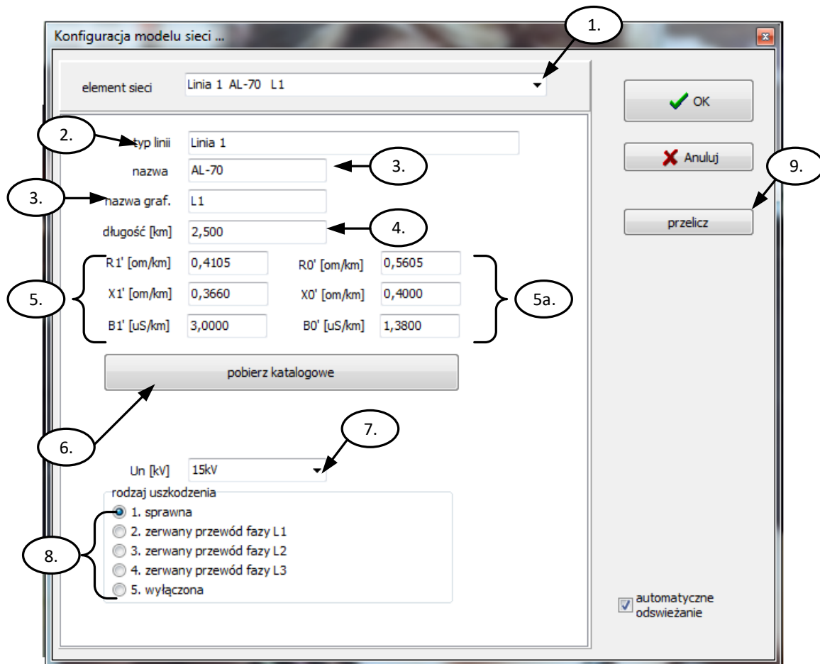
Rys.8.7. Okno edycji parametrów modelu linii
