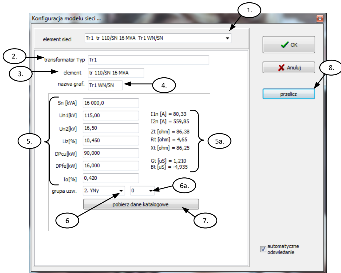
Rys.8.6. Okno edycji parametrów transformatora
